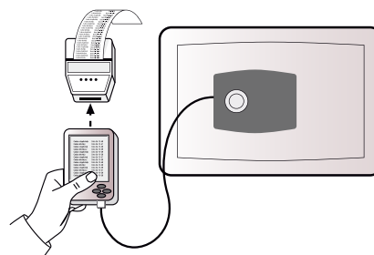
PRESA USB. STORICO DELLE ULTIME 100 OPERAZIONI, VISUALIZZABILE ATTRAVERSO CEU UNIT E DISPLAY. USB PLUG. AUDIT TRAIL OF THE LAST 100 OPERATIONS READABLE THROUGH CEU DEVICE AND DISPLAY.
